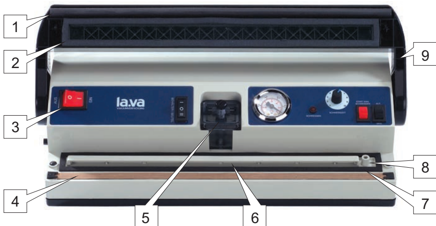
Hauptbestandteile Maschinen: V.100® / V.200® / V.300®
